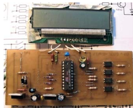
Рис. 4. Печатная плата и индикатор
